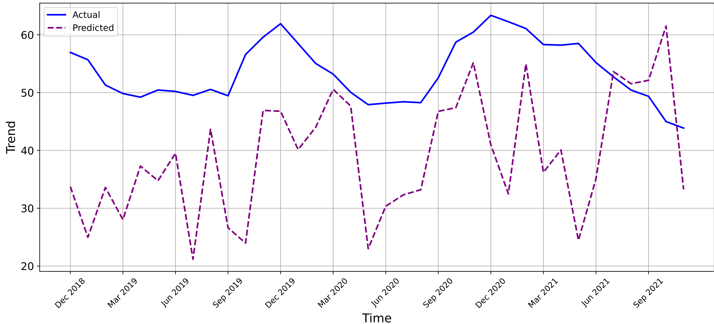
Mentions-MITM - Validation
